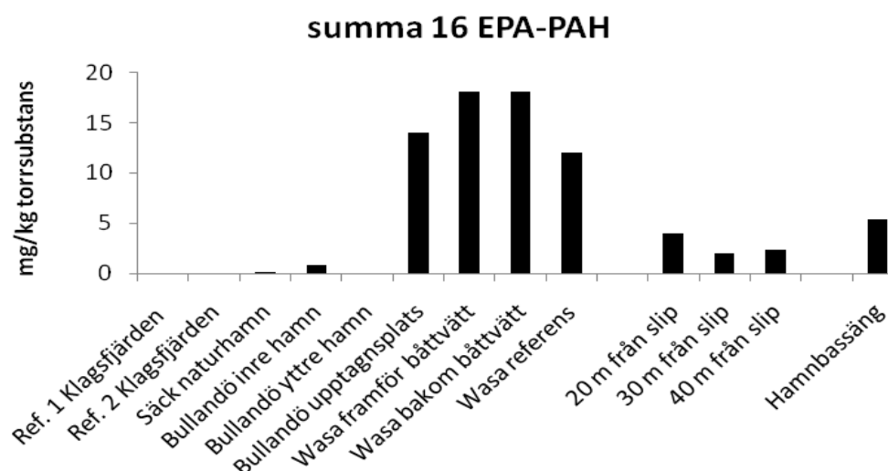
Figur 3. Den sammanlagda halten av de 16 vanligaste polyaromatiska föreningarna (PAH) i ytsediment från olika typer av hamnområden visas i figuren.
