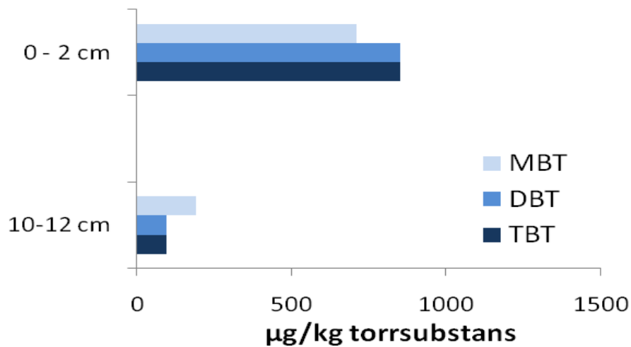
Figur 2 B. Halter av organiska tennföreningar i ytsediment 40 m från båtupptagningsplatsen i en marina på Djurgården i Stockholm, 2007.
