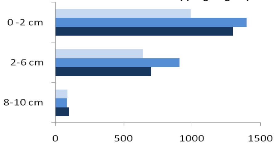
Figur 2A. Halter av organiska tennföreningar i ytsediment 20 m från båtupptagningsplatsen i en marina på Djurgården i Stockholm, 2007.
