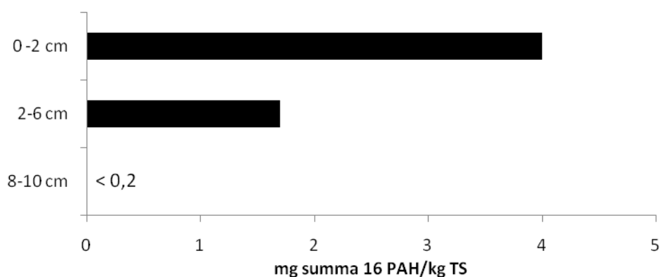
Figur 5A. Den sammanlagda halten av de 16 vanligaste polyaromatiska föreningarna (PAH) i sediment från olika djup på en station 20 m utanför en slip i en marina i inre del av Stockholm visas i figuren.
