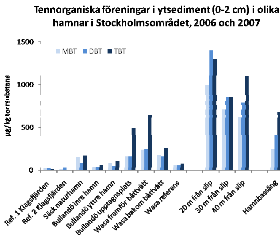
Figur 1. Halter av tennorganiska föreningar i ytsediment från olika typhamnar i Stockholmsområdet.
