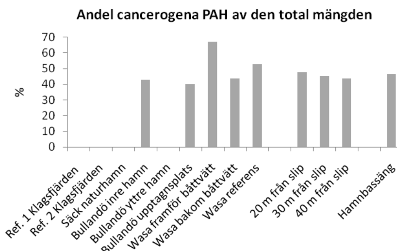
Figur 4. Den procentuella andelen av cancerogen polyaromatiska kolväten visas i figuren.
